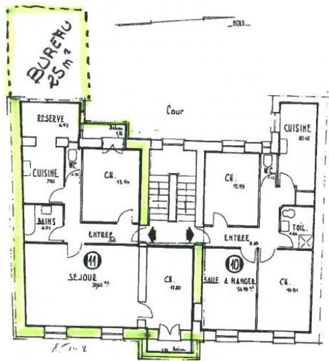
1er ETAGE
