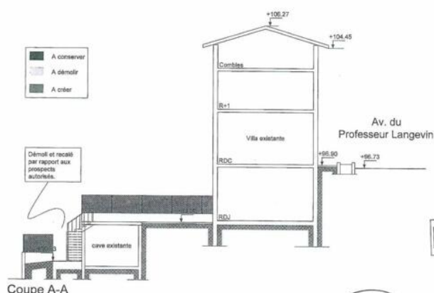
Coupe A-A
