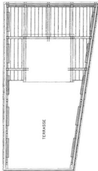
VUE EN PLAN DU PERGOLAT PROJET
