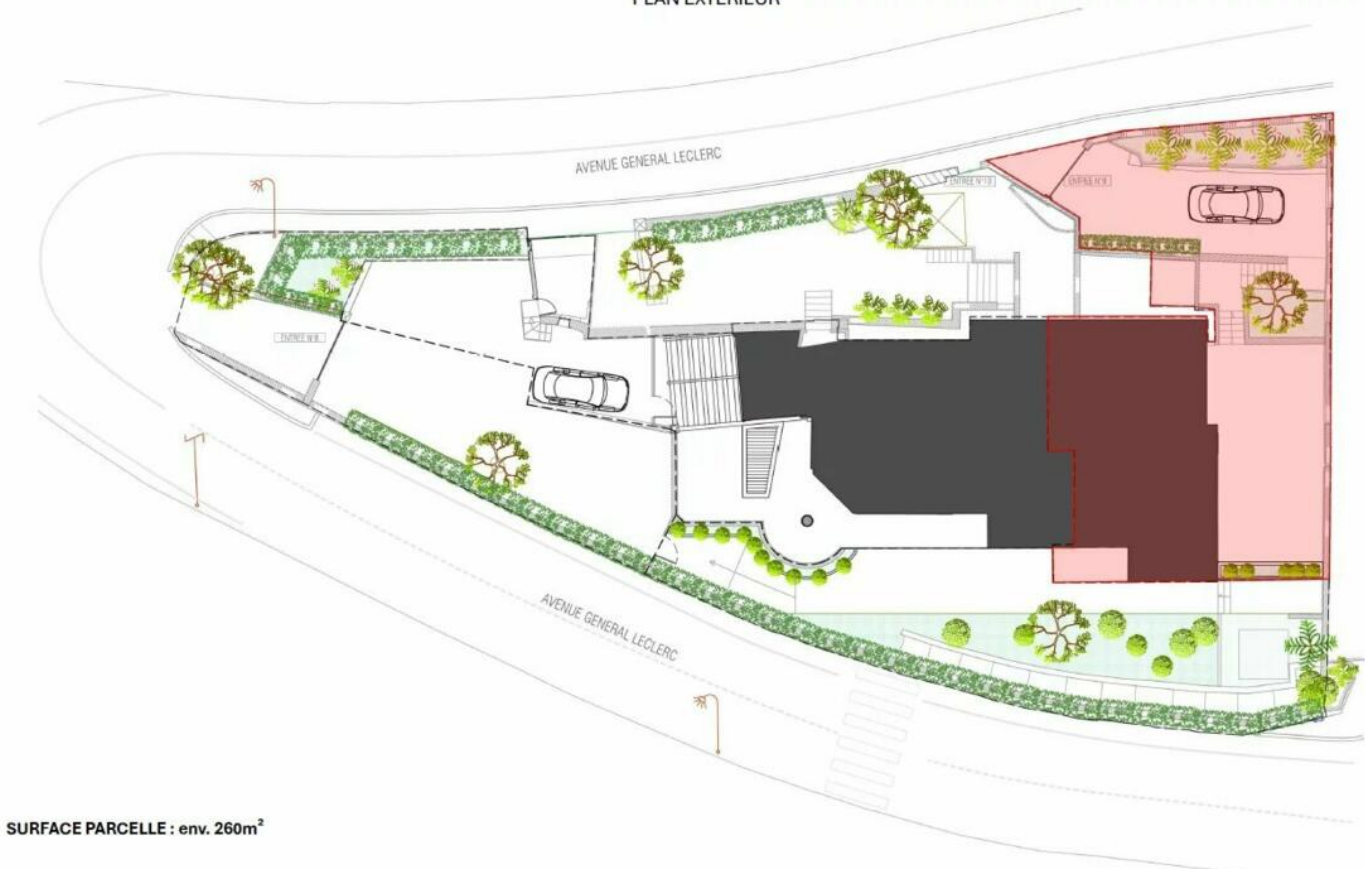
PLAN EXTERIEUR
