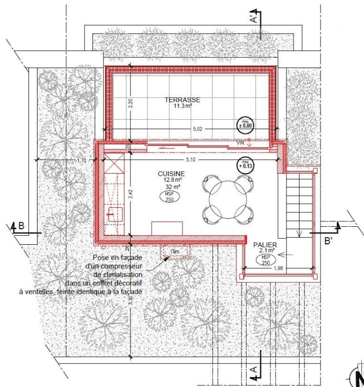
PLAN TOITURE - TERRASSE
